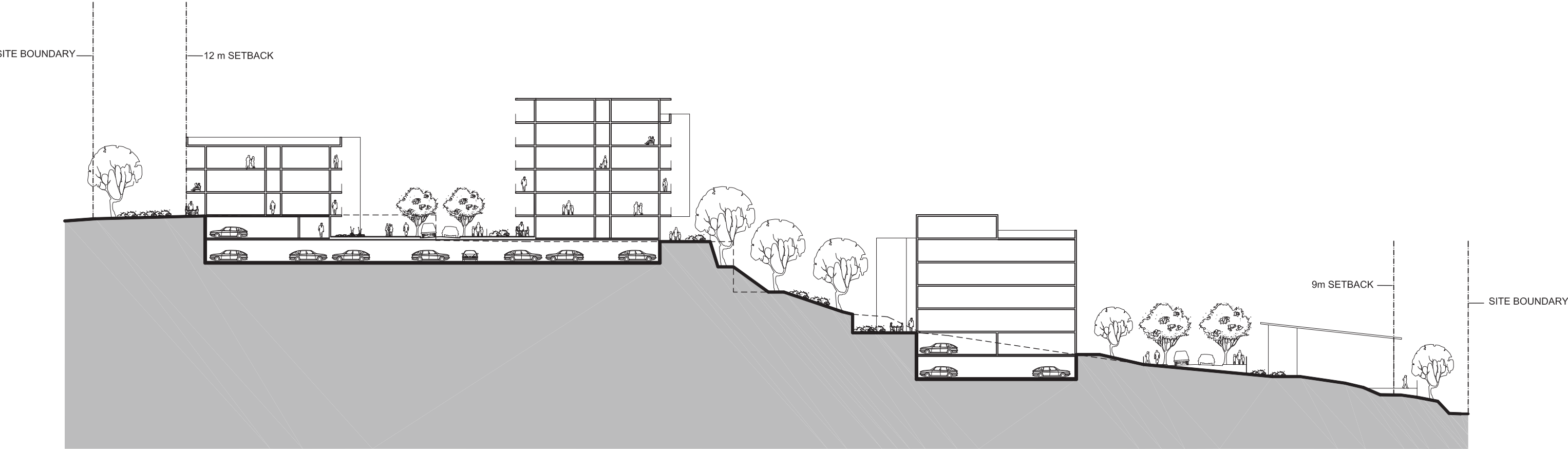
Section A-A
