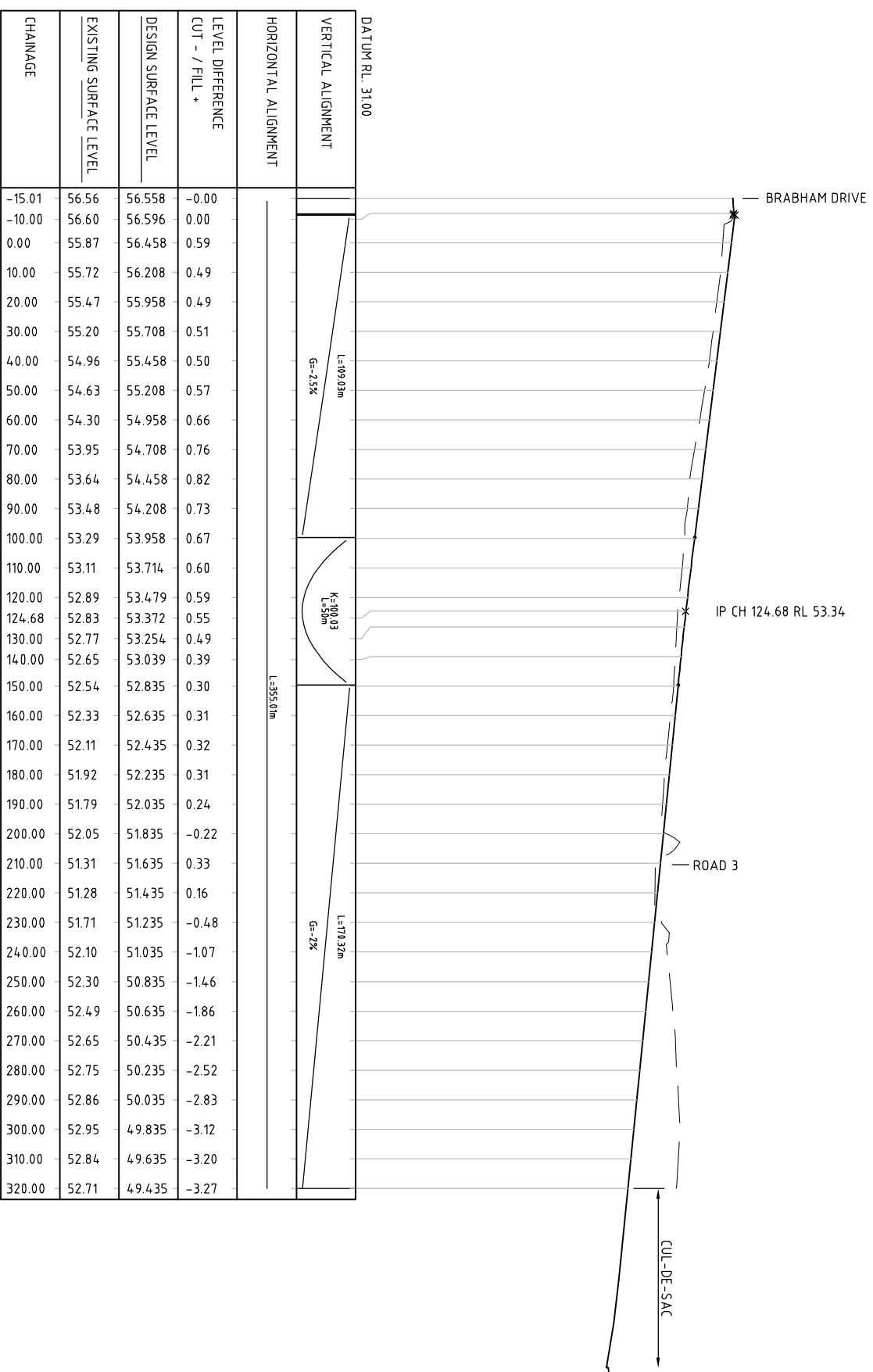
LONGITUDINAL SECTION - ROAD 4 HORZ 1:1000 VERT 1:200
