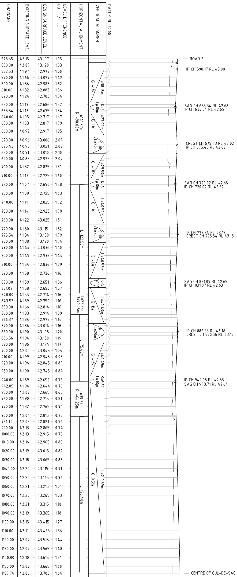
LONGITUDINAL SECTION - ROAD 5 HORZ 1:1000 VERT 1:200
