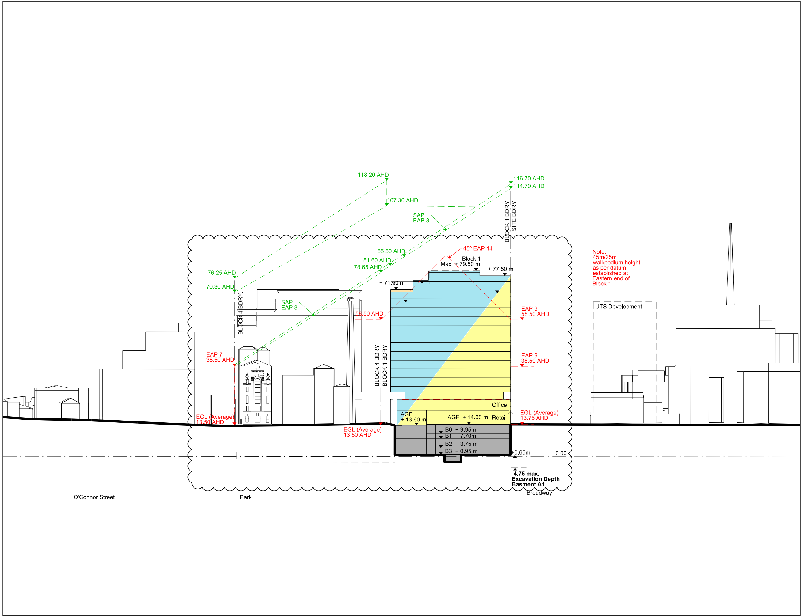
01 Section 02 1:1000
