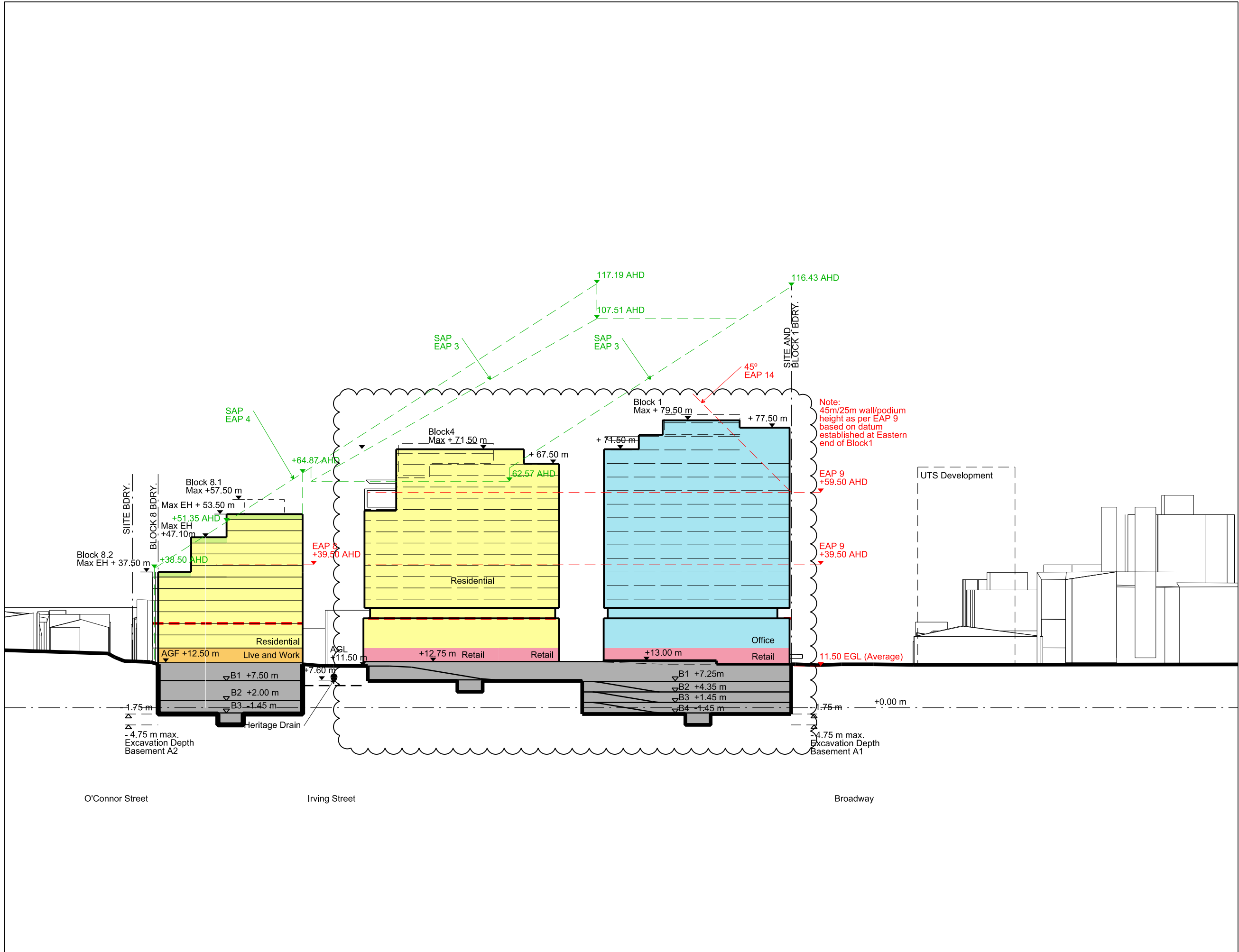
01 Section 01 1:1000
