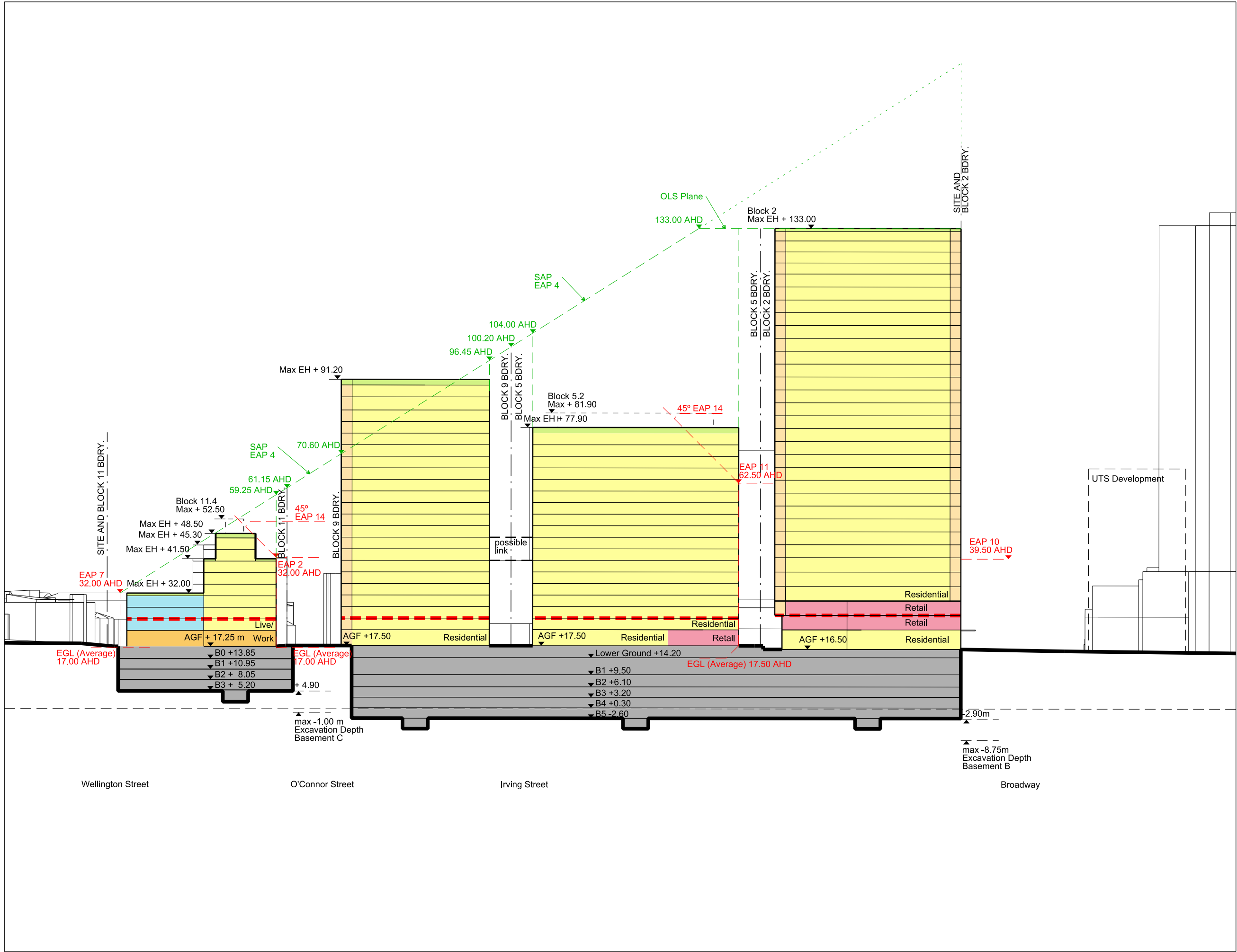
01 Section 03 1:1000
