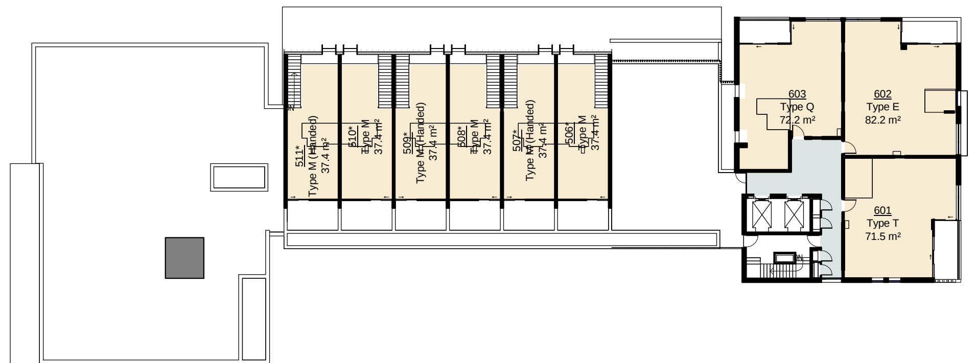
8 Level 6 1 : 300
