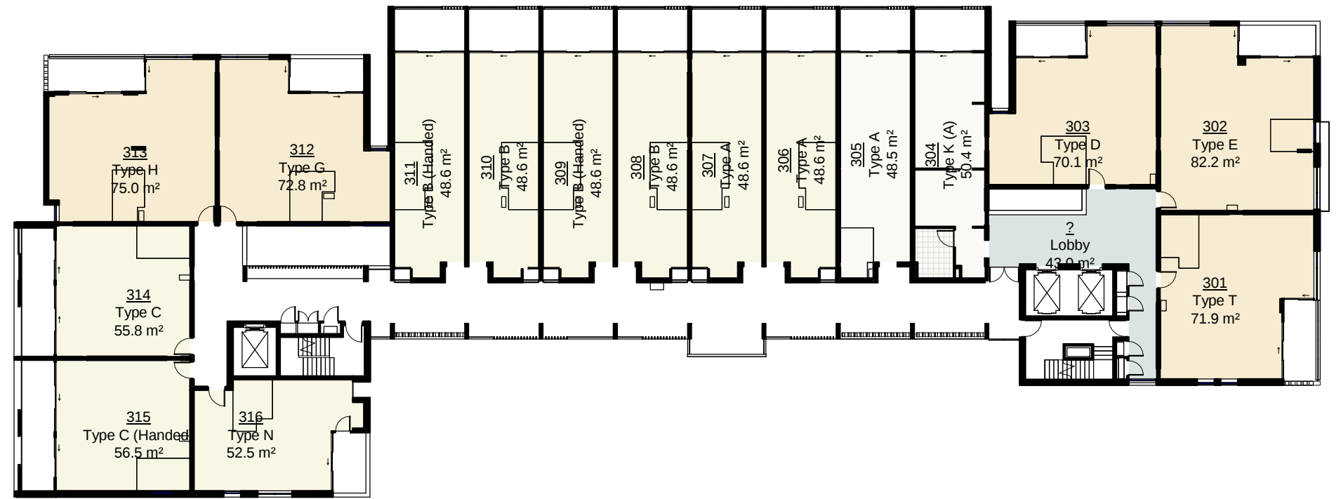
5 Level 3 1 : 300
