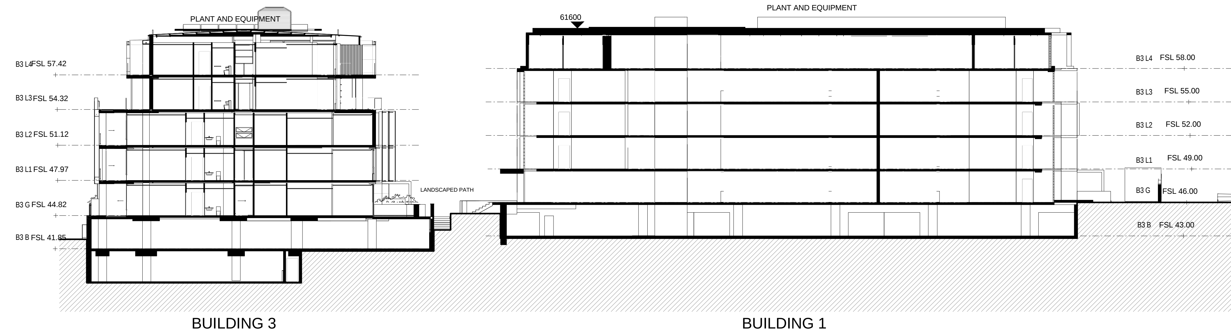
2 SECTION 2 1 : 200
