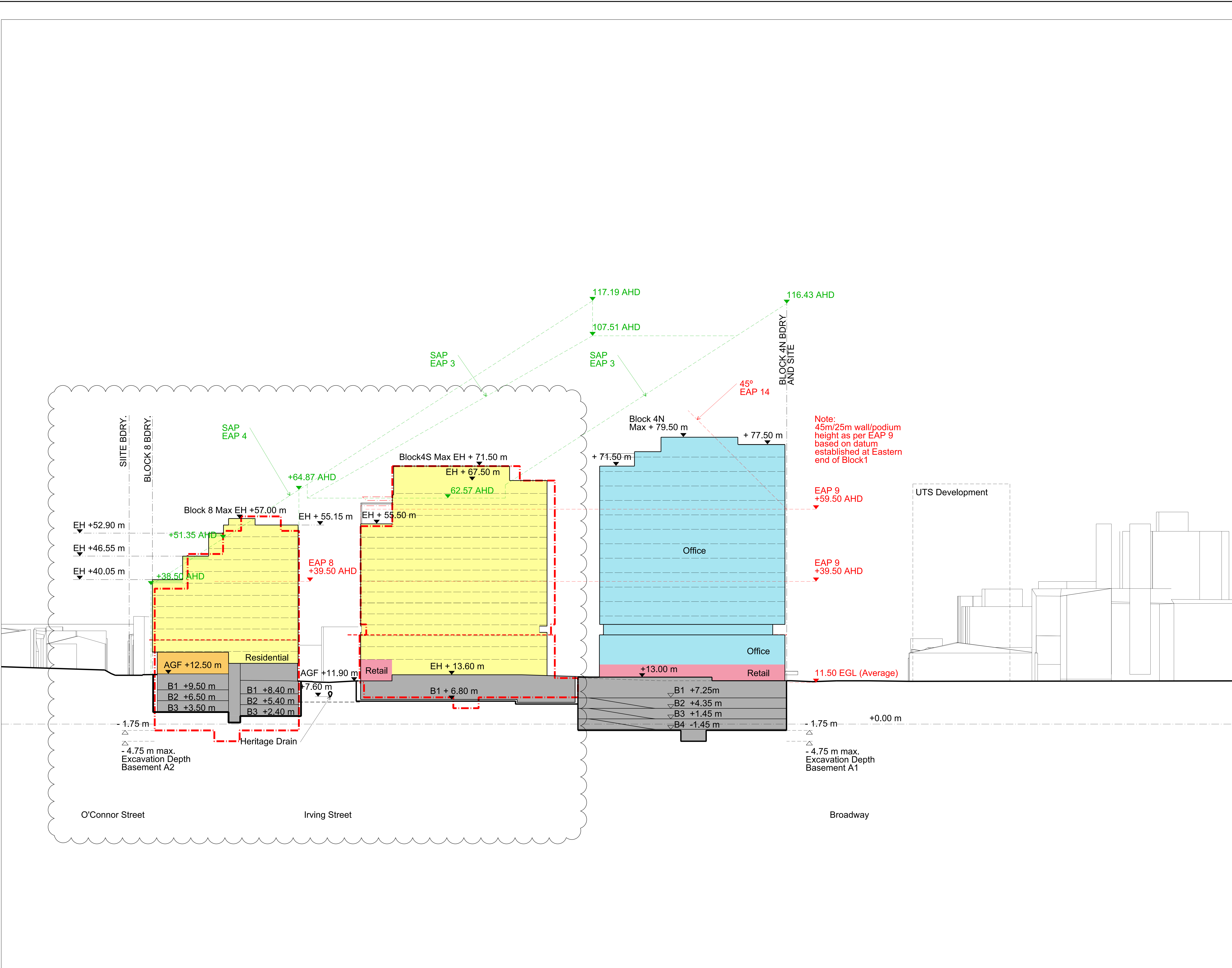
01 Section 01 1:1000
