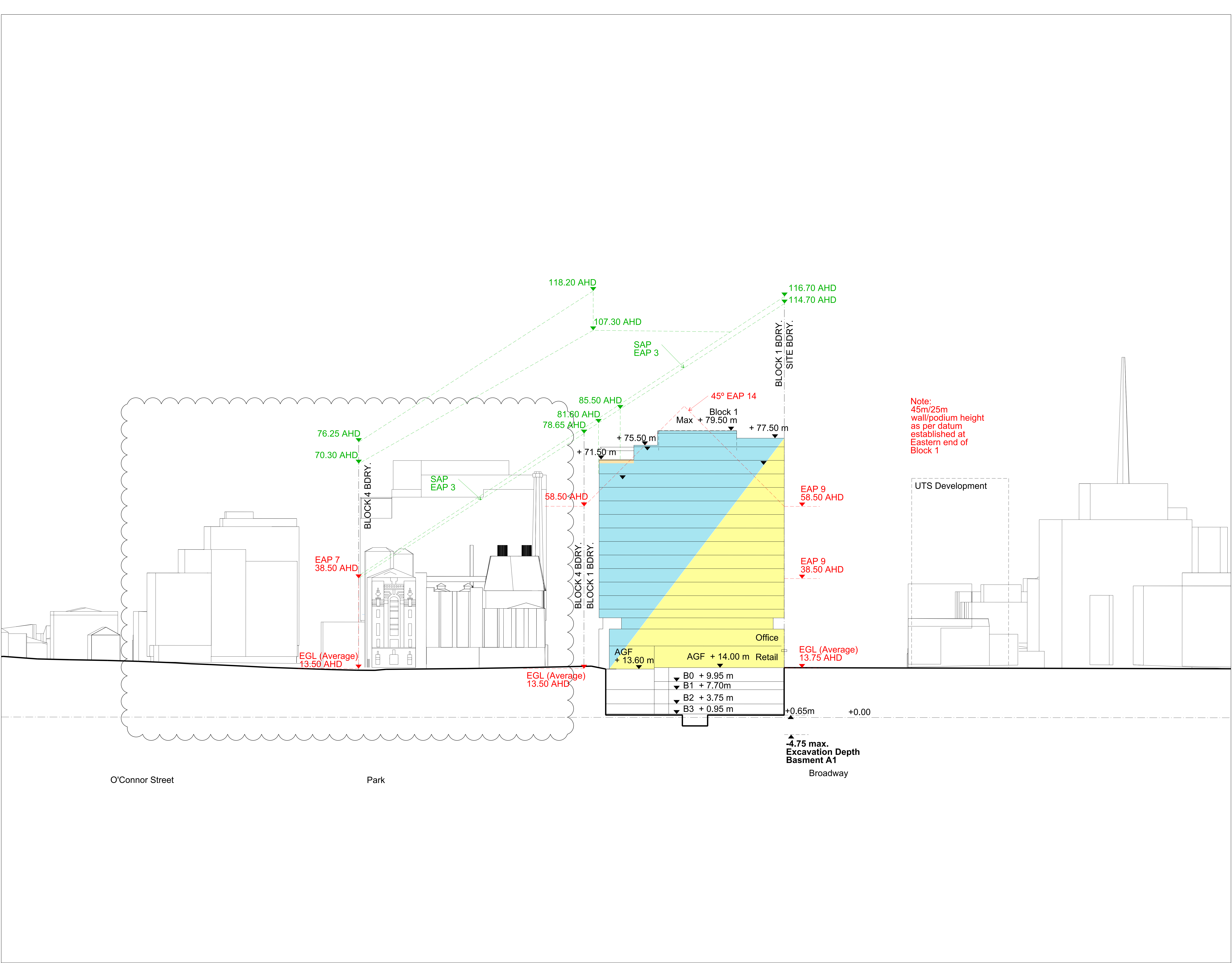
01 Section 02 1:1000
