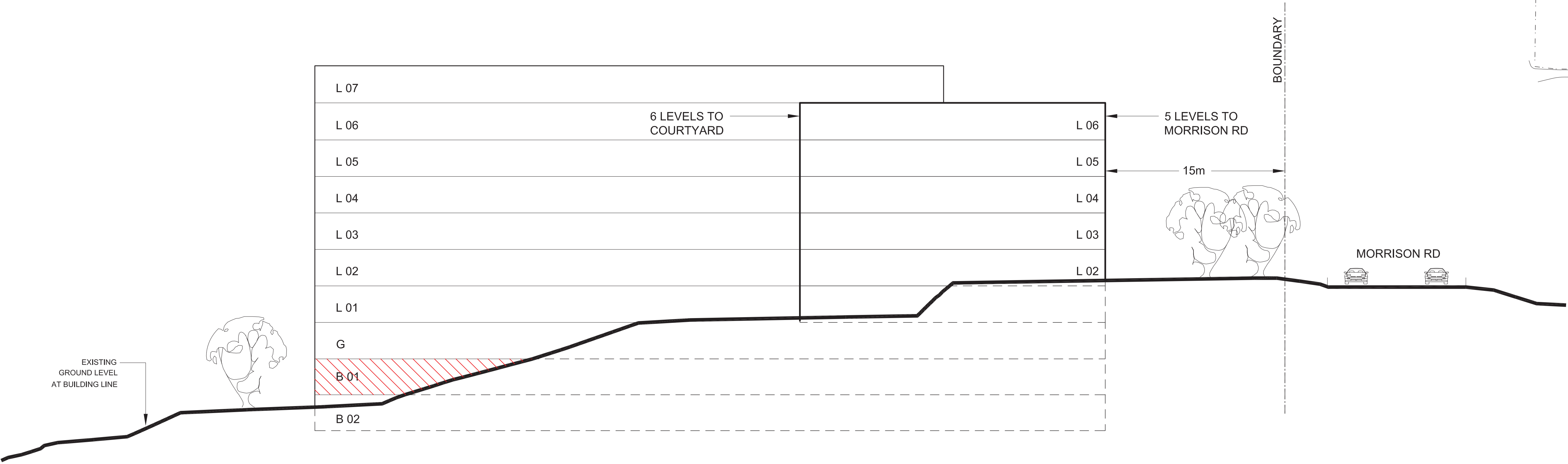
Section DD
