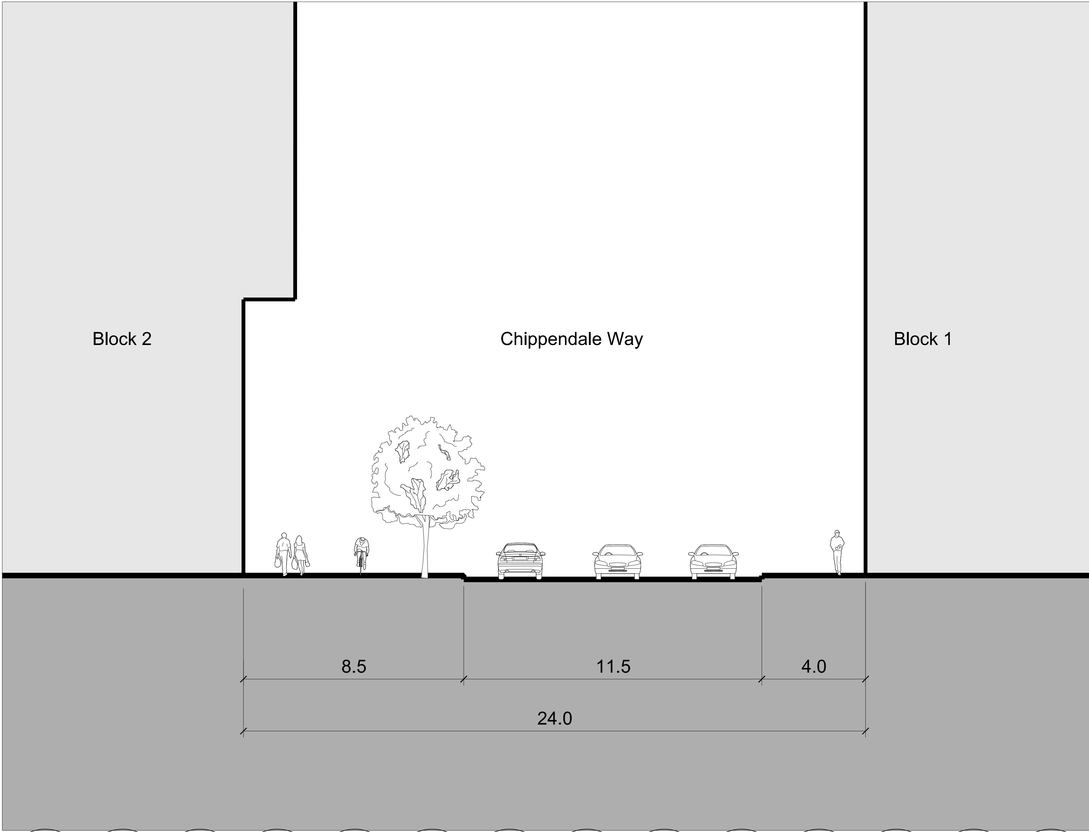
01 Section 1:250
