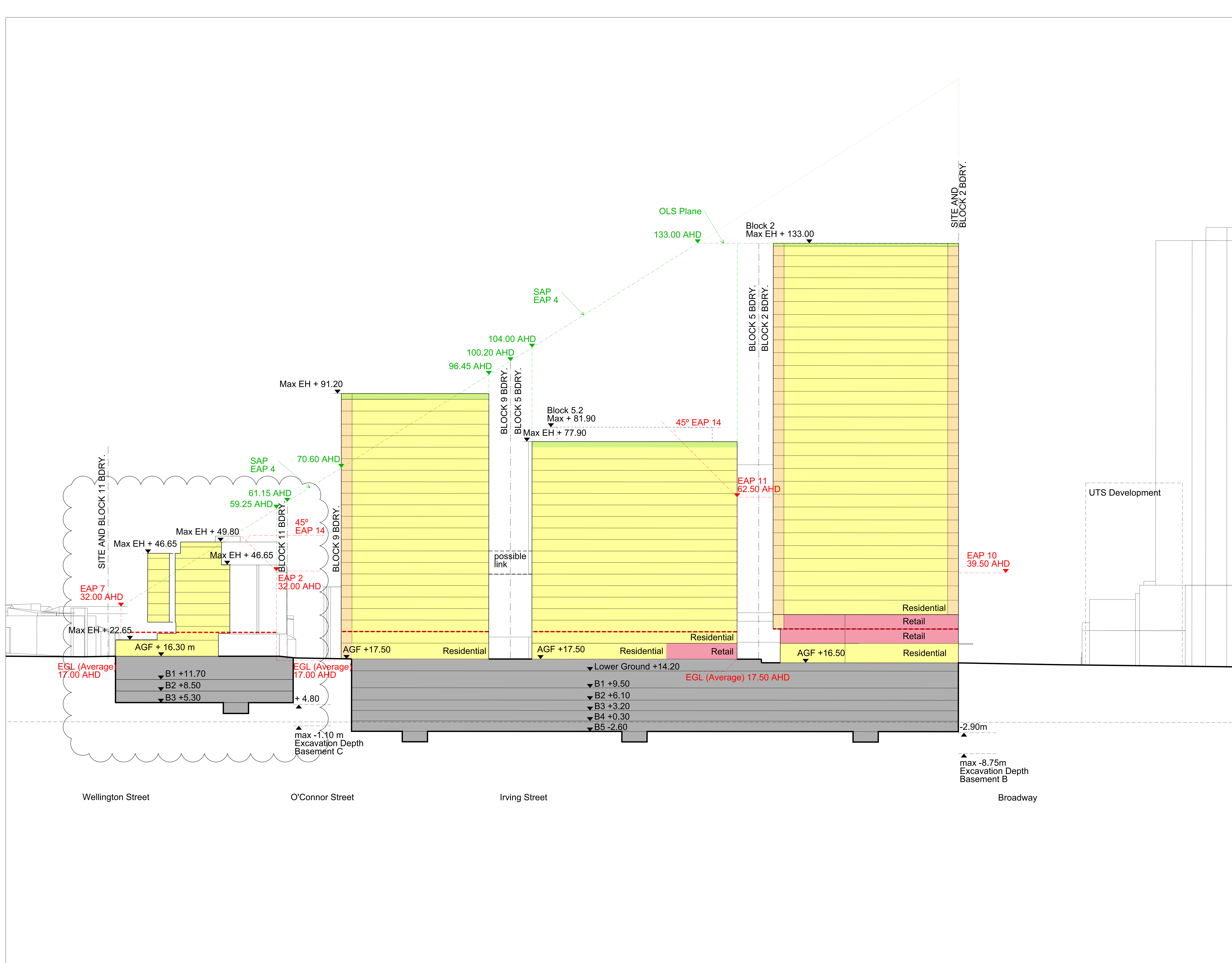
01 Section 03 1:1000
