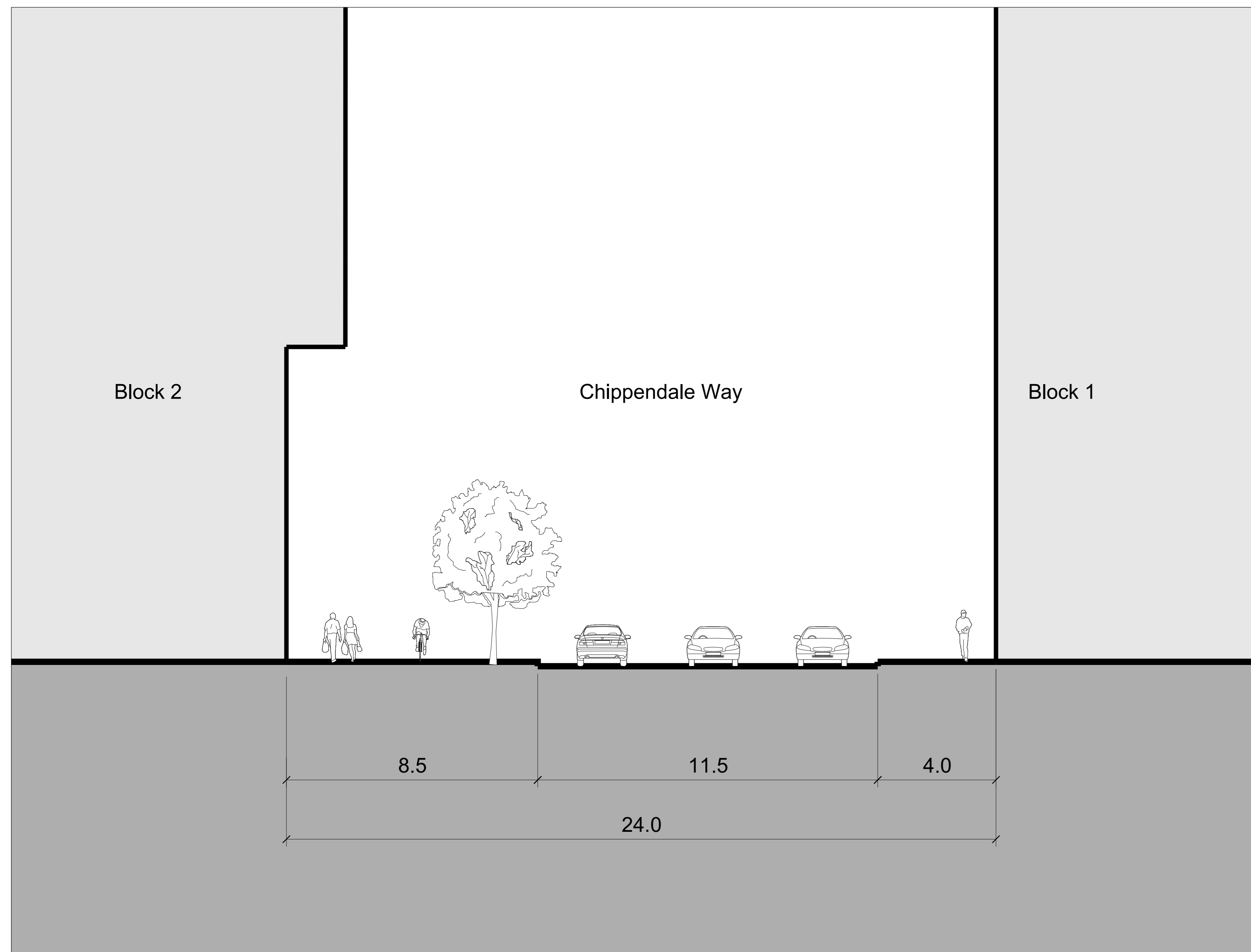
01 Section 1:250
