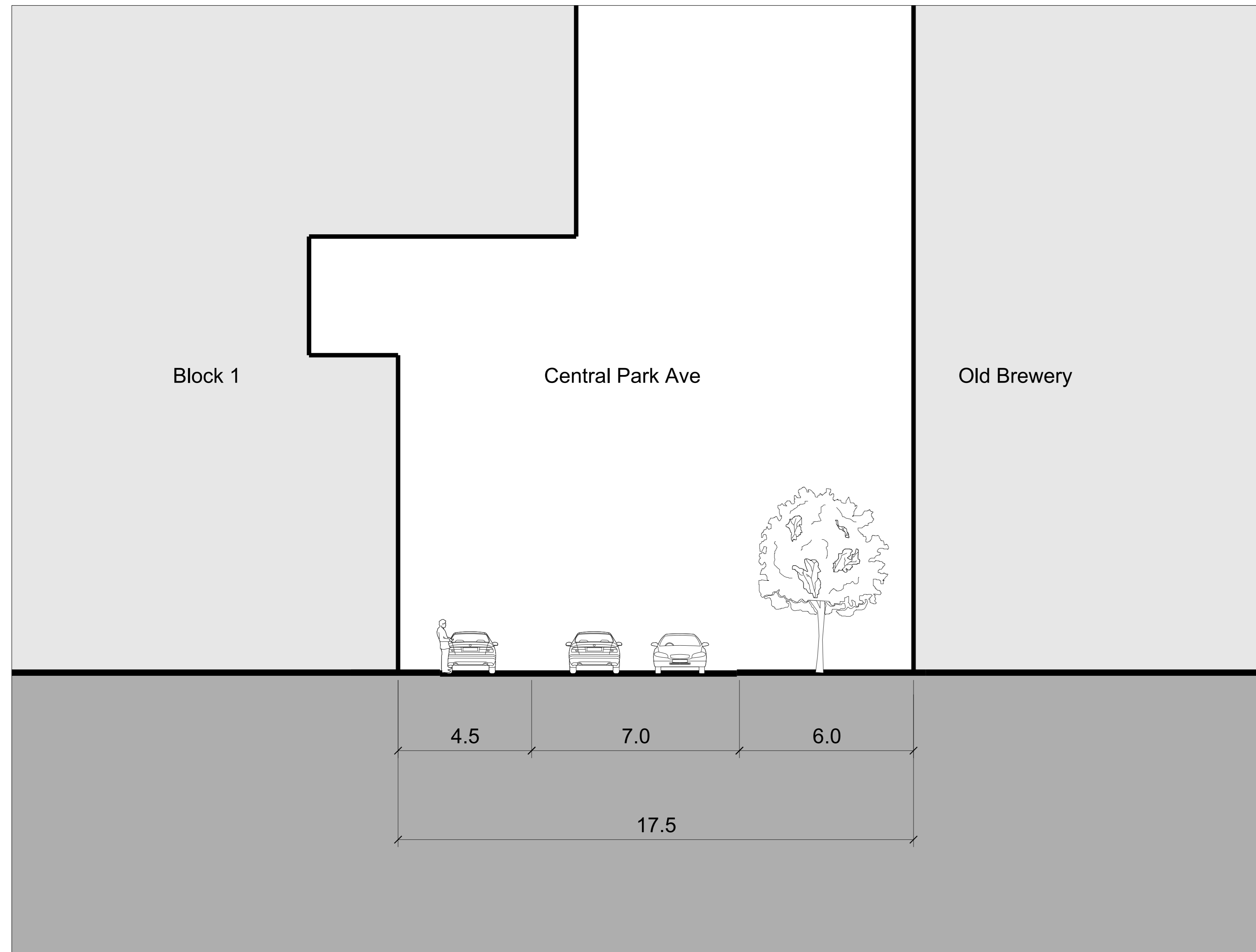
03 Section 1:250
