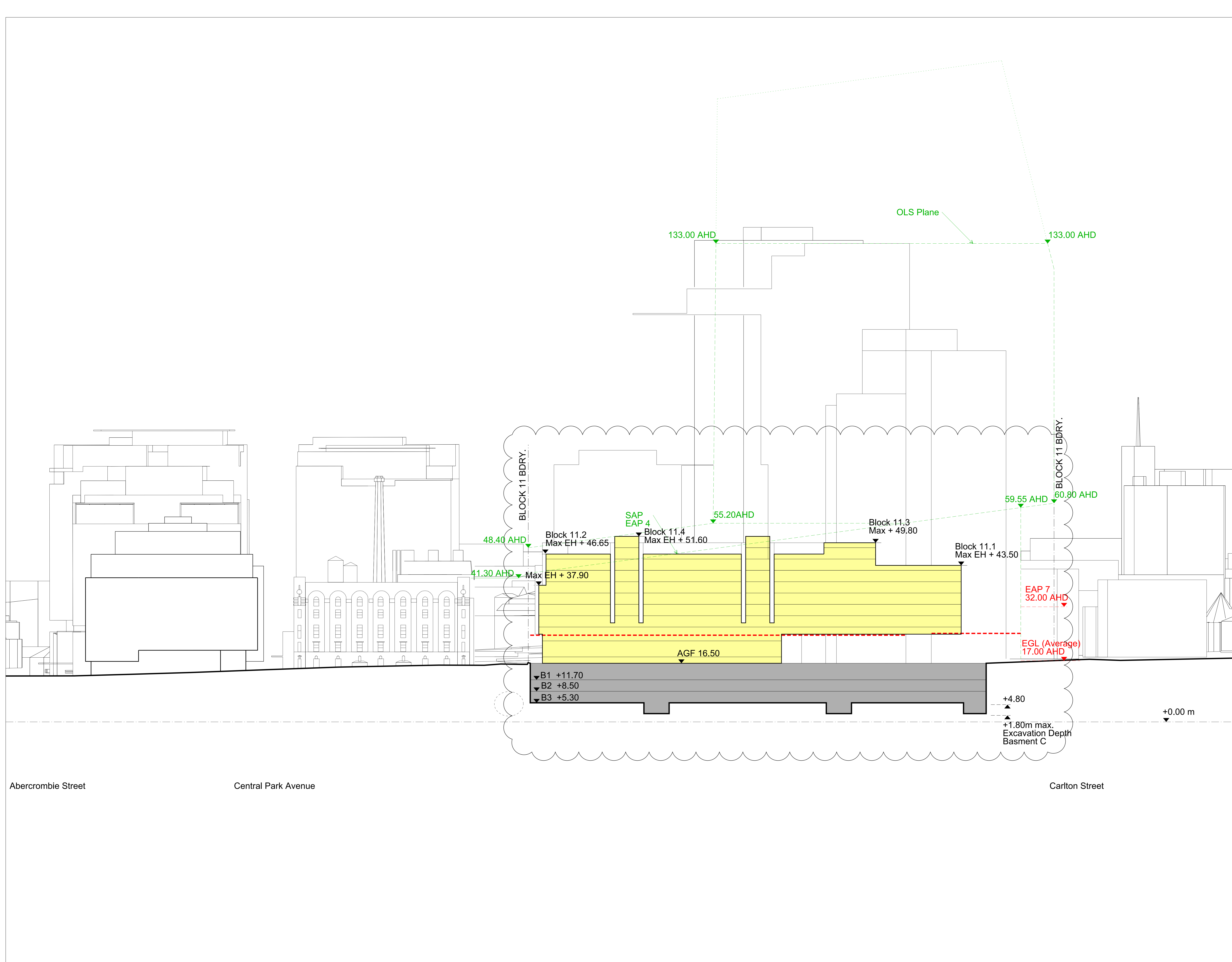
01 Section 07 1:1000
