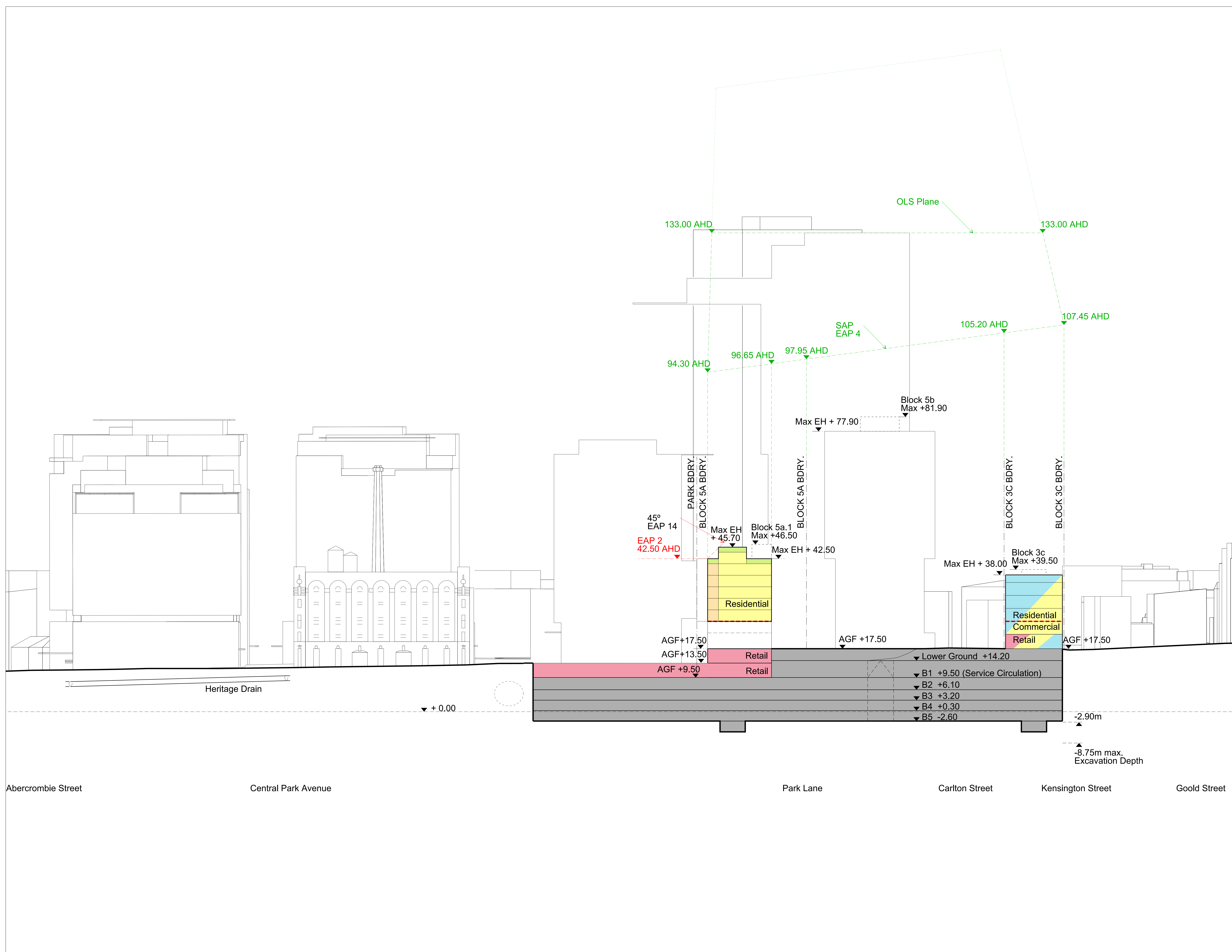
01 Section 06 1:1000
