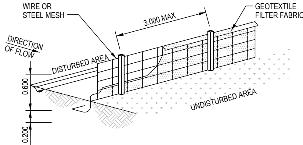
SEDIMENT FENCE SCALE: N.T.S.
