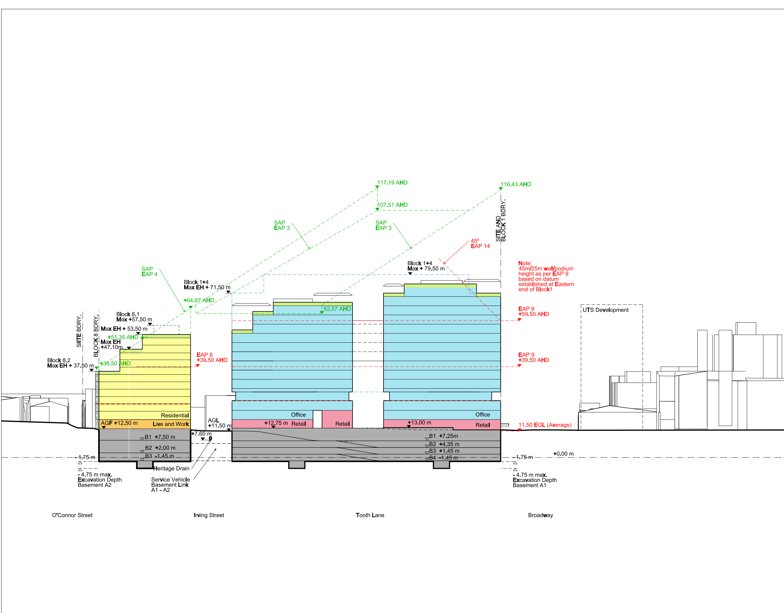
01 Section 01 1:1000
