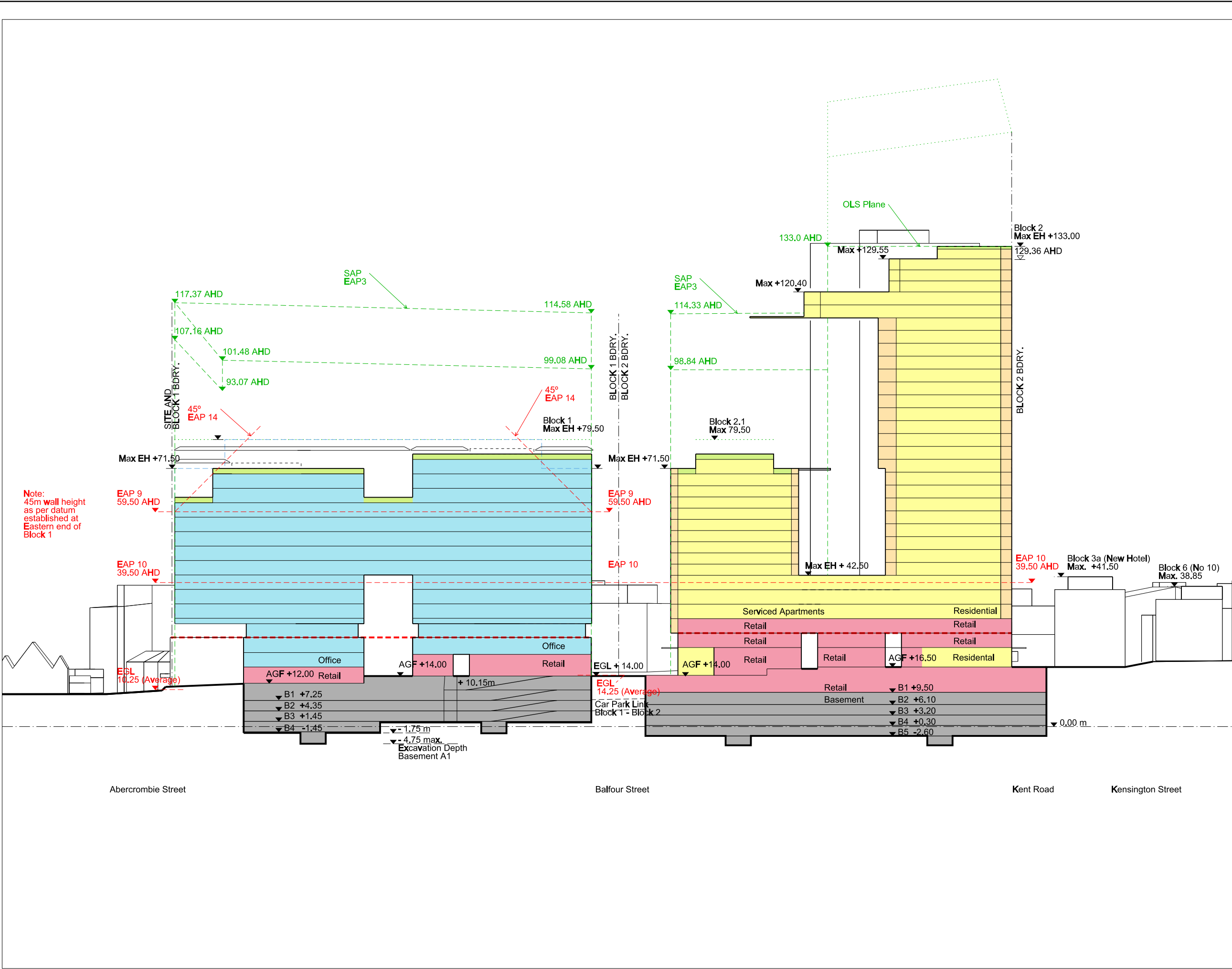
01 Section 04 1:1000
