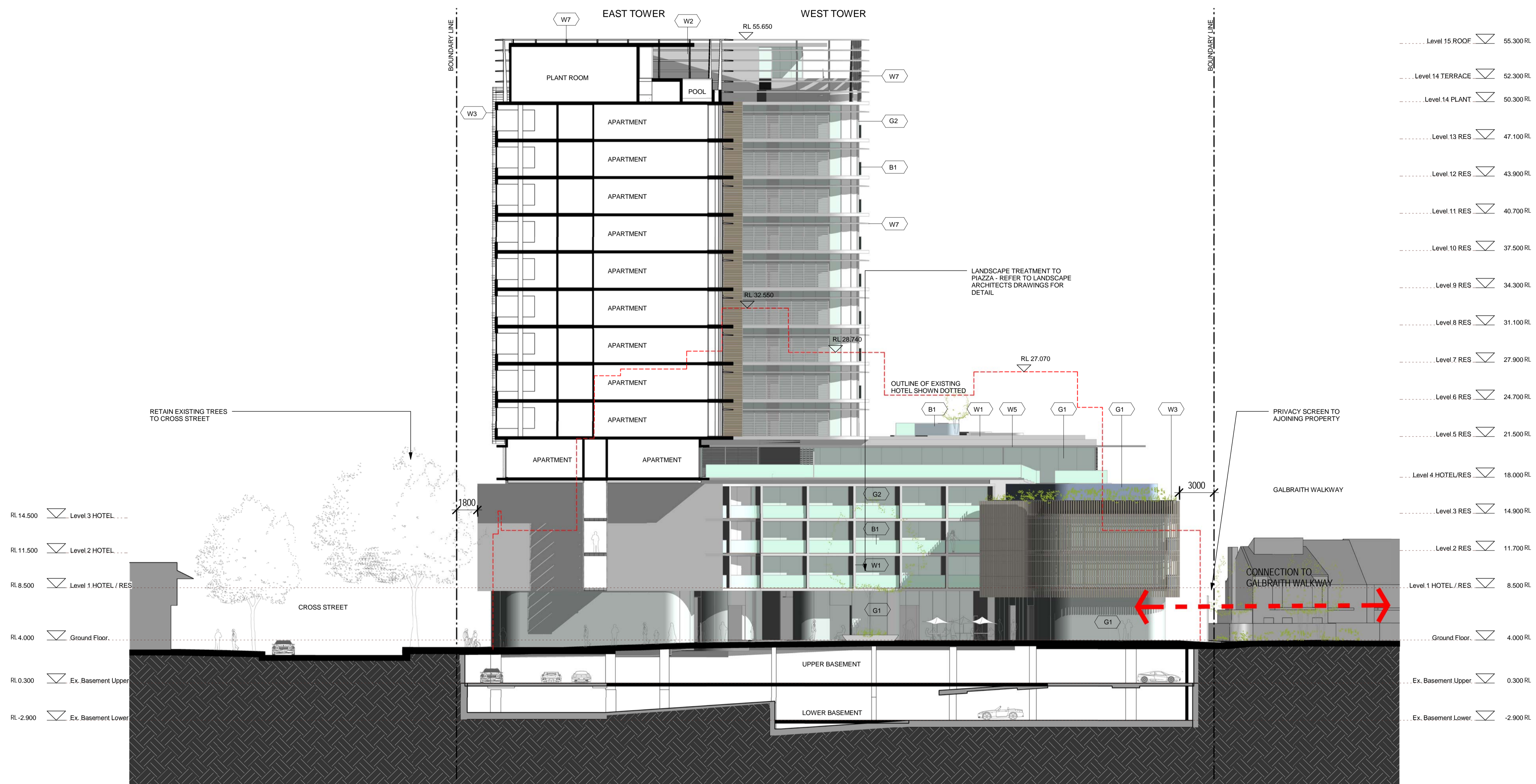
1 Section D-D Scale: 1 : 200
