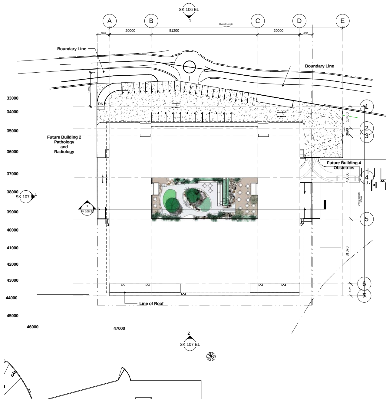
1 Site 1 : 500
