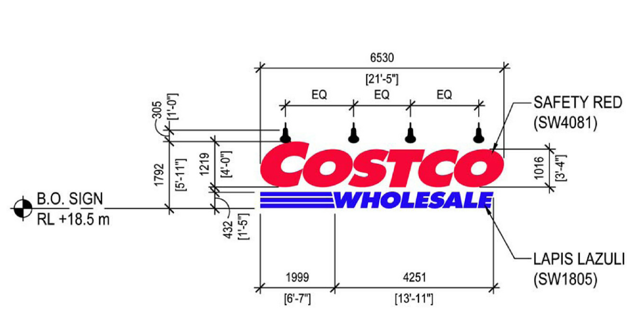
A MAIN ENTRY SIGNAGE SCALE: 1:100
