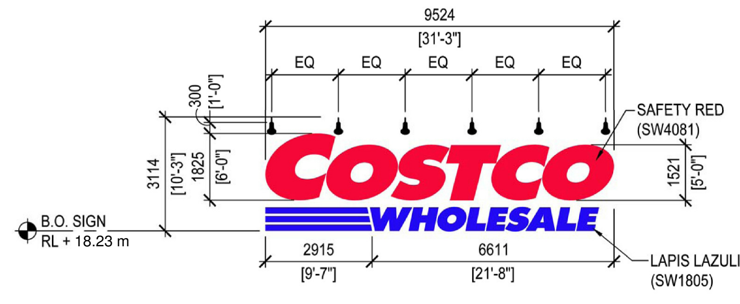
B MAIN ENTRY SIGNAGE SCALE: 1:100
