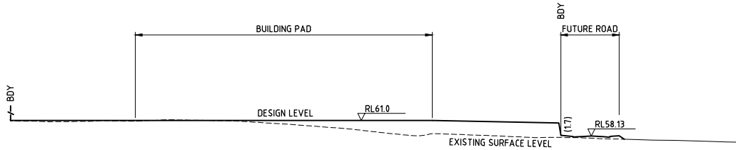
SECTION 6 Scale: 1:1000(H) 1:500(V)
