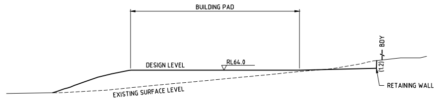
SECTION 2 Scale: 1:1000(H) 1:500(V)
