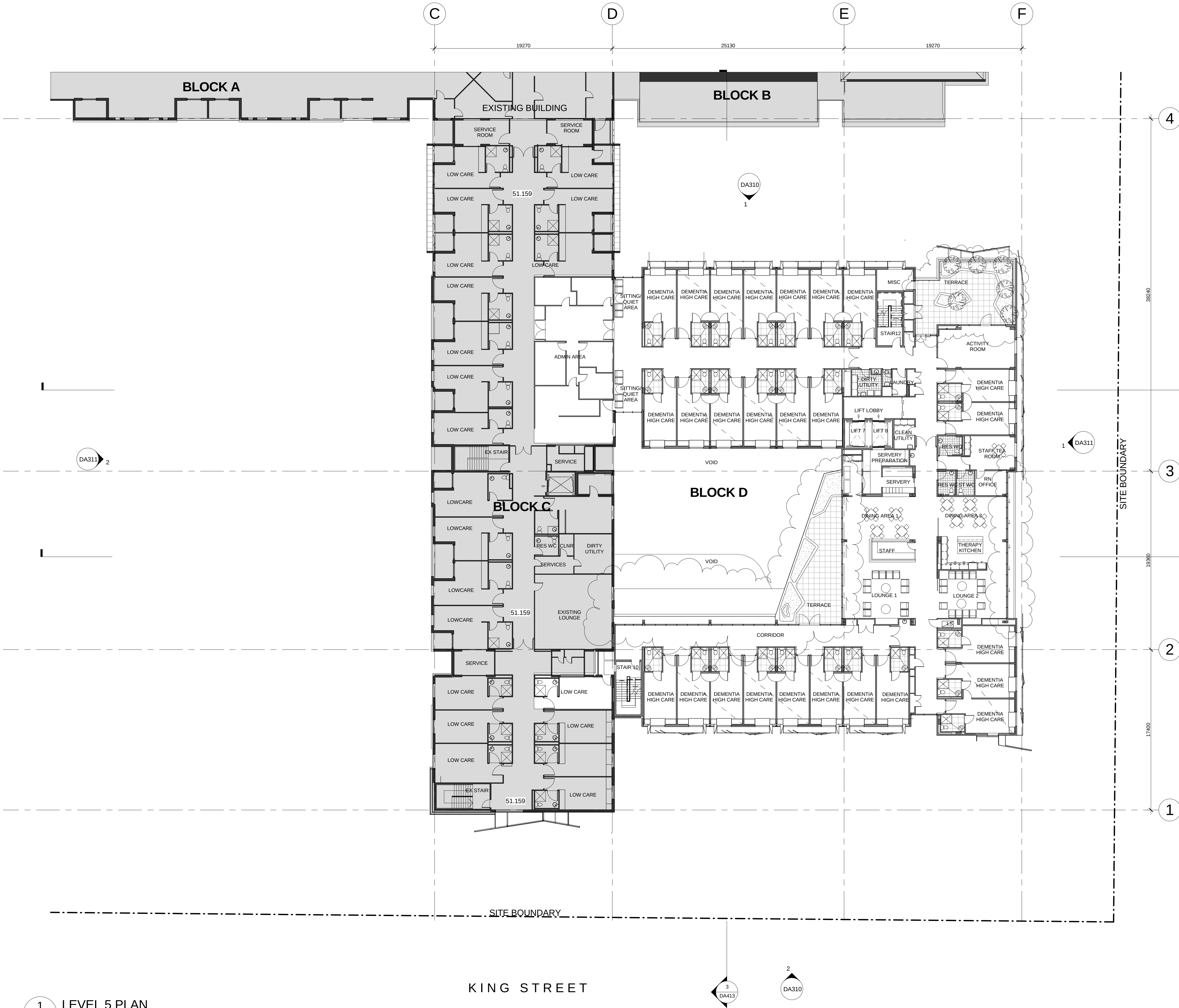
1 LEVEL 5 PLAN A056 1:200
