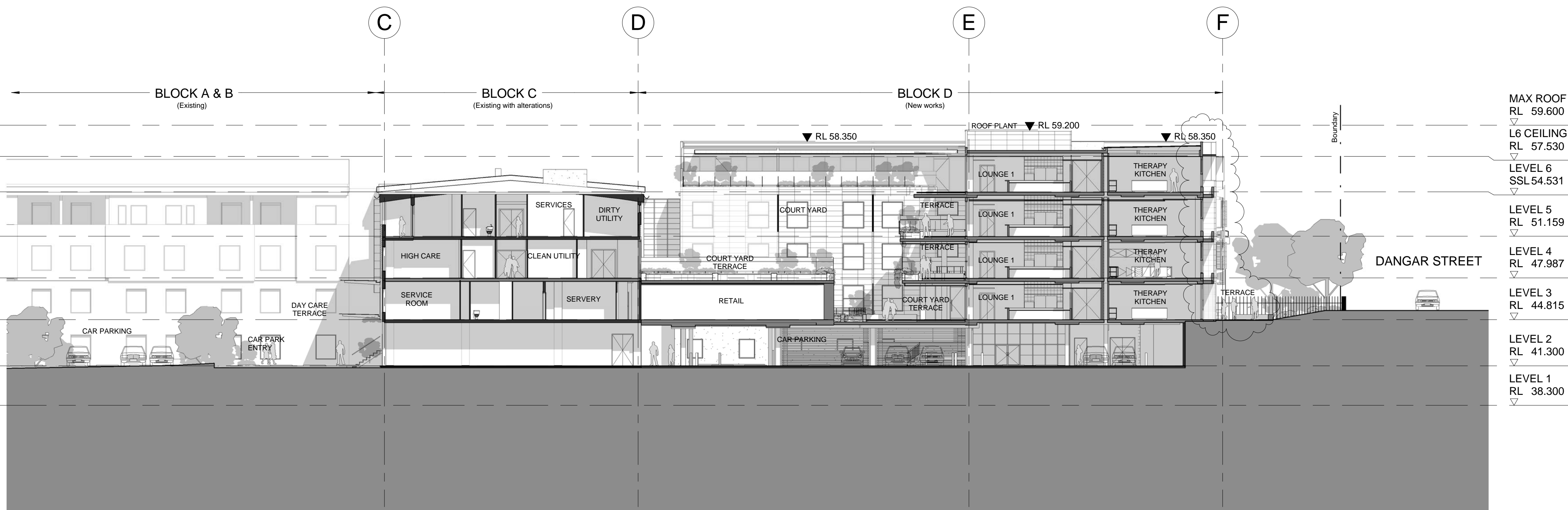
1 SECTION A023 1 : 200
