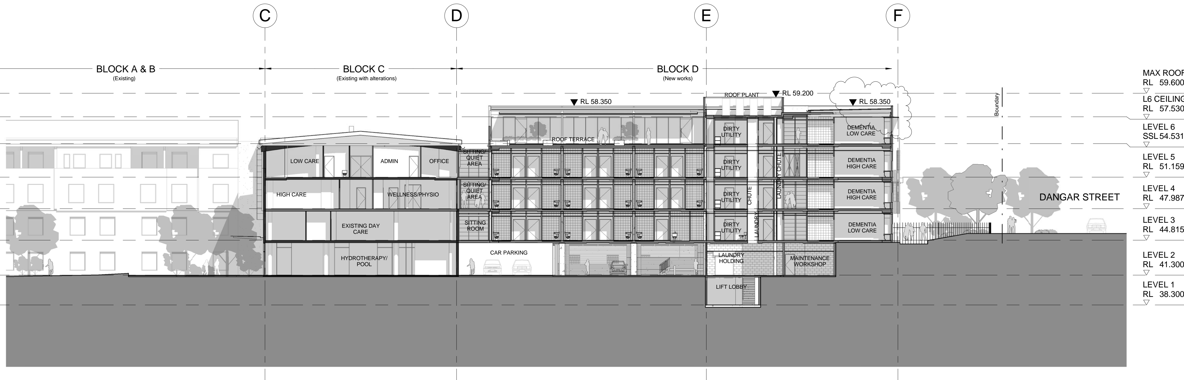
2 SECTION A023 1 : 200
