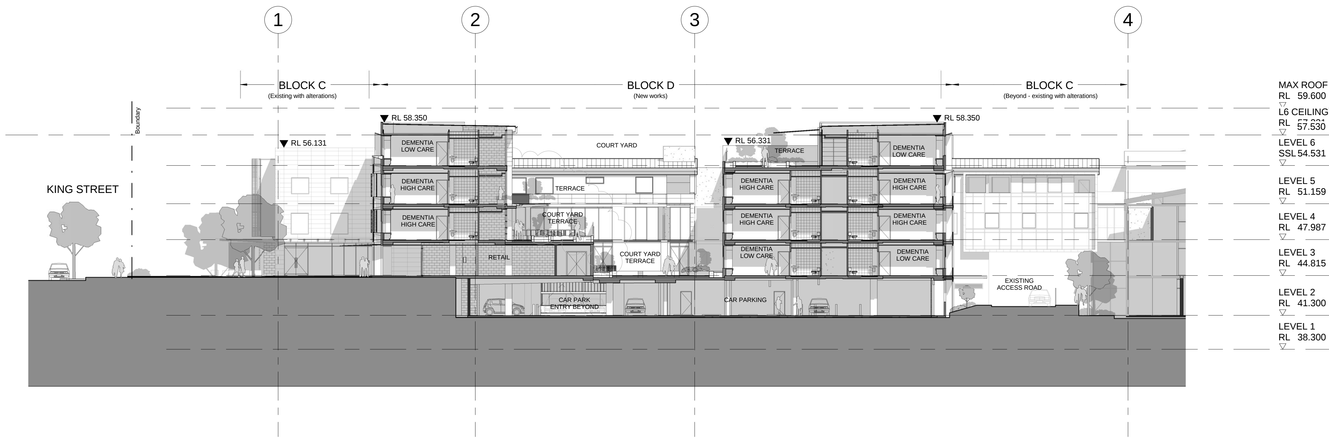
3 SECTION A204 1 : 200
