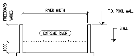
3 TYP. RIVER SECTION 1 : 100
