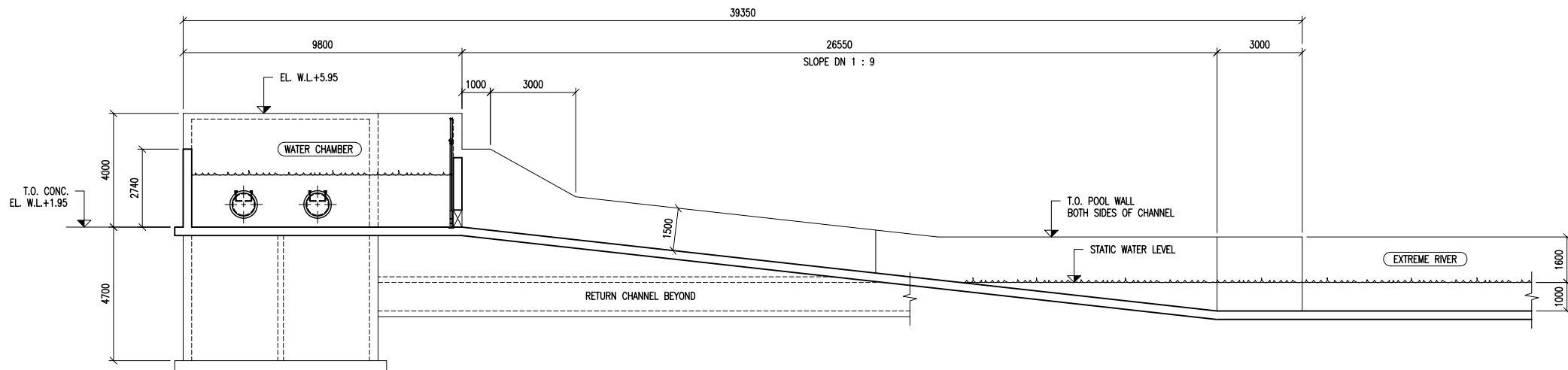
2 SECTION 1 : 100
