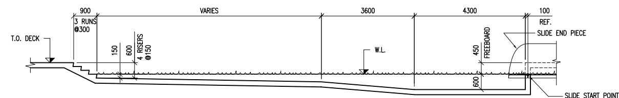
3 POOL SECTION 1 : 75
