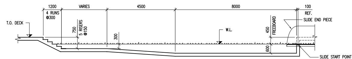
2 POOL SECTION 1 : 75
