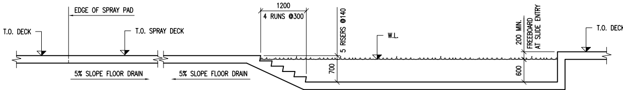
2 POOL SECTION — 1 : 50
