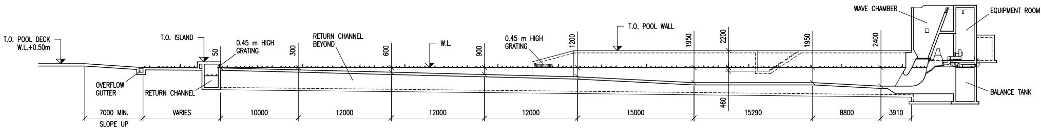
2 SURF WAVE POOL SECTION W800 1 : 250
