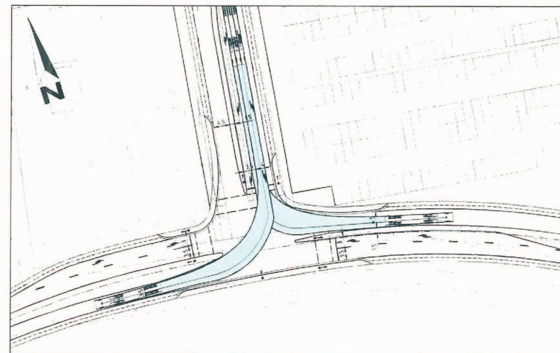
CONSTRUCTION VEHICLE 19M AV TURN B AND D
