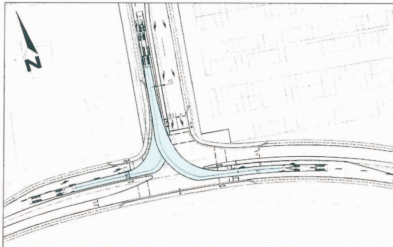
CONSTRUCTION VEHICLE 19M AV TURN A AND C
