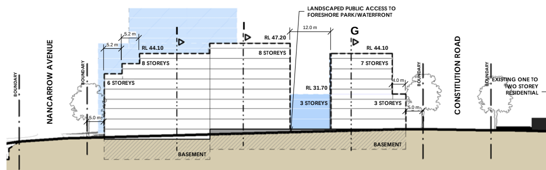
4. Elevation 2 EA004-A 1 : 500
