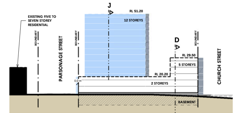
3 5. Elevation 3 EA005-A 1 : 500
