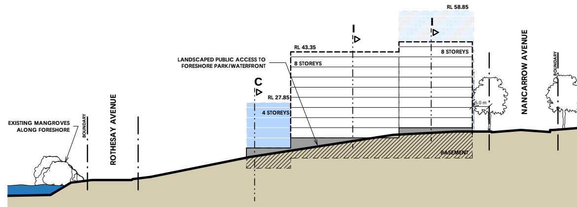
6. Elevation 1 1 : 500
