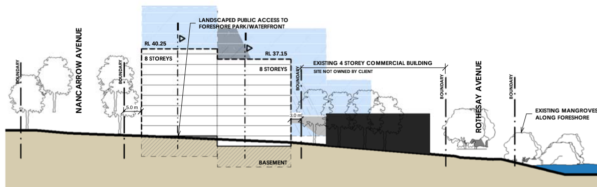
6. Elevation 2 1 : 500
