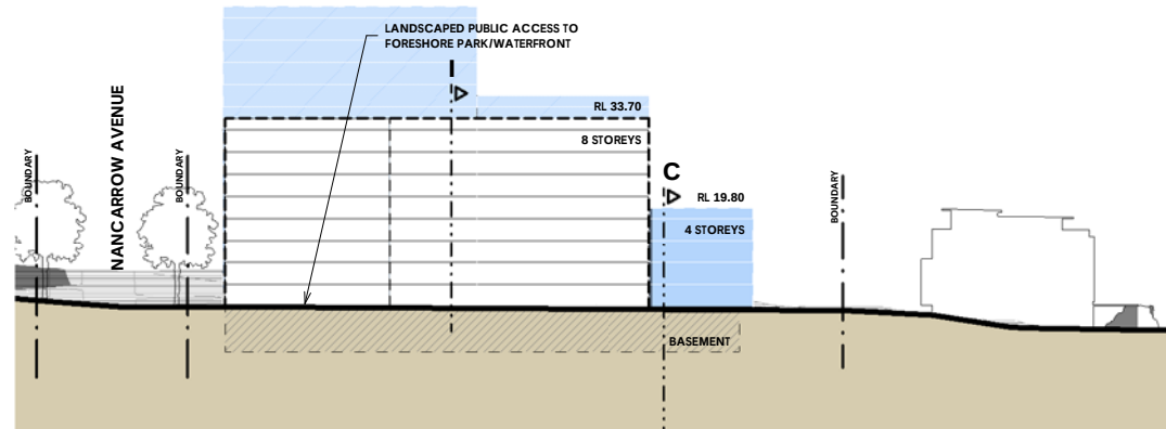
1 7. Elevation 1 EA007-A 1 : 500
