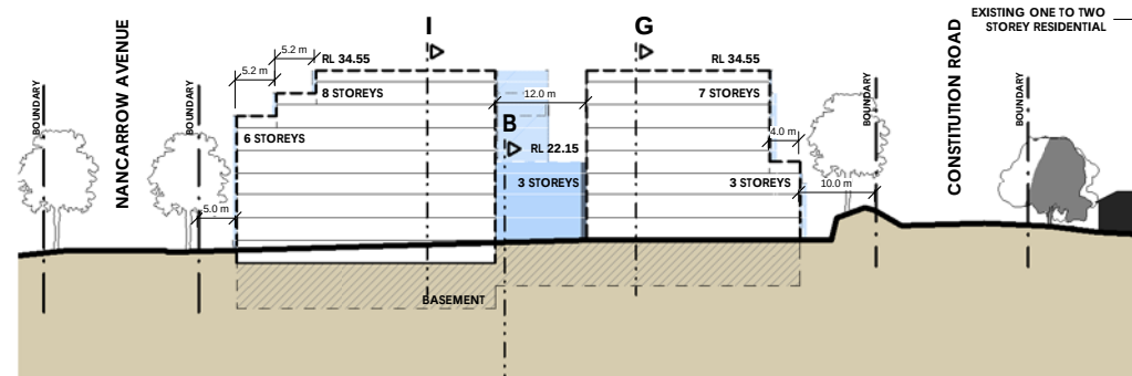
1 8. Elevation 1 EA008-A 1 : 500
