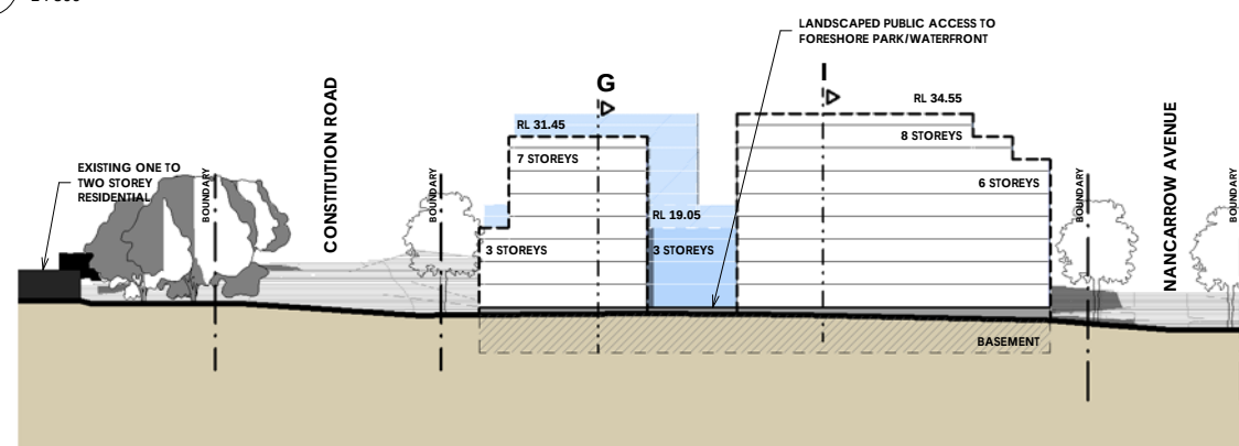
2 8. Elevation 2 EA008-A 1 : 500
