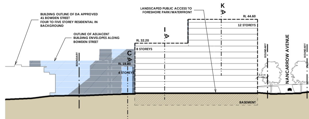
9. Elevation 1 1 : 500
