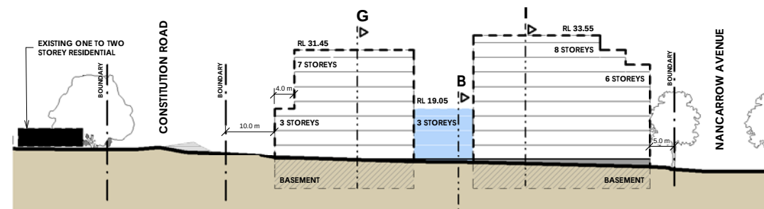
2 10. Elevation 2 1 : 500
