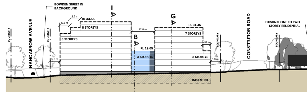
1 10. Elevation 1 1 : 500
