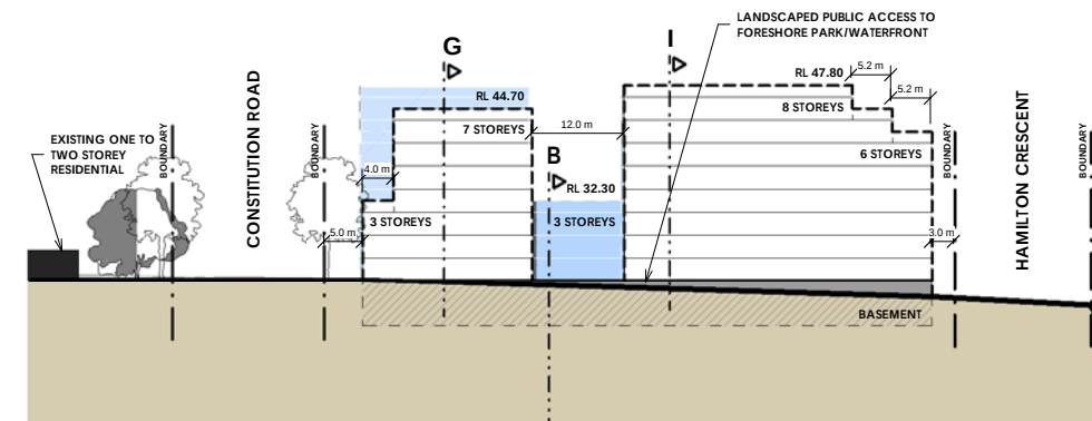
2. Elevation 2 EA002-A 1 : 500
